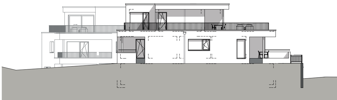
Südwest-Fassade
