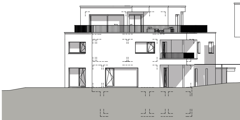
Nordwest-Fassade
