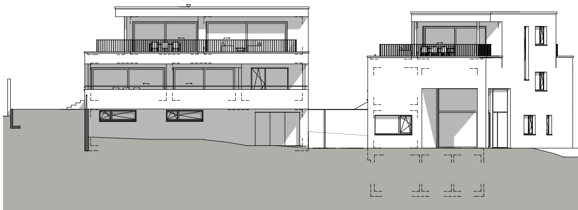
Südost-Fassade
