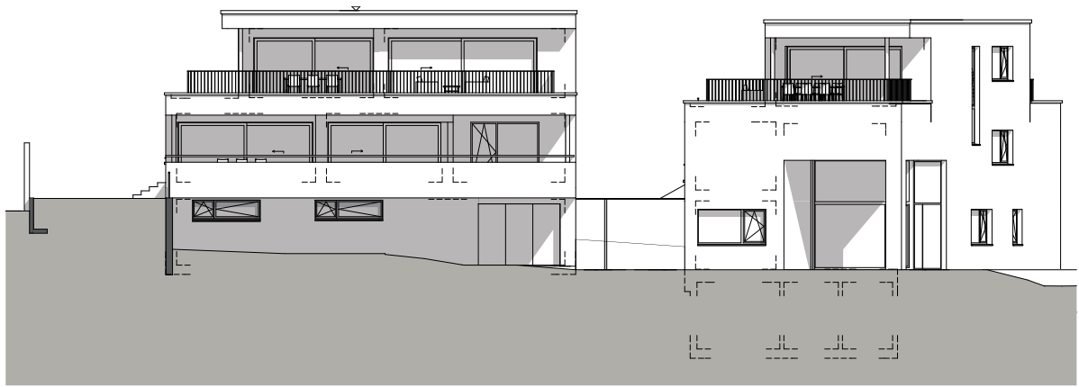
Südost-Fassade
