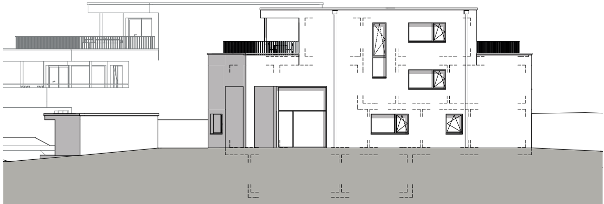
Ost-Fassade
