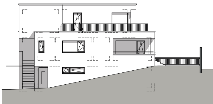
Nordwest-Fassade
